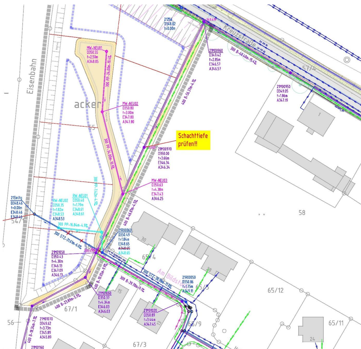
Abb. 1: (Auszug aus der Fachplanung Lageplan Kanal (Lageplan), Ingenieurbüro Falkenhahn & Partner, Stand Mai 2020)
